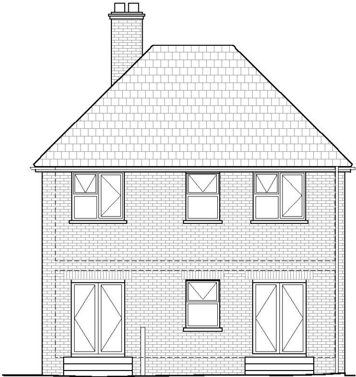
Elevation 3
