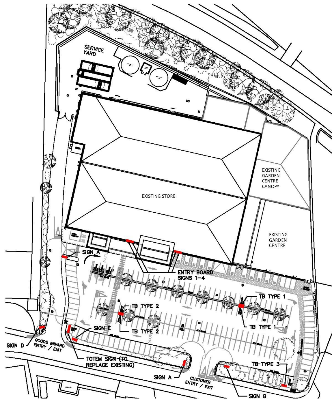
SITE PLAN 1:1000
