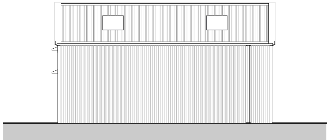
FLANK (N-W) ELEVATION
