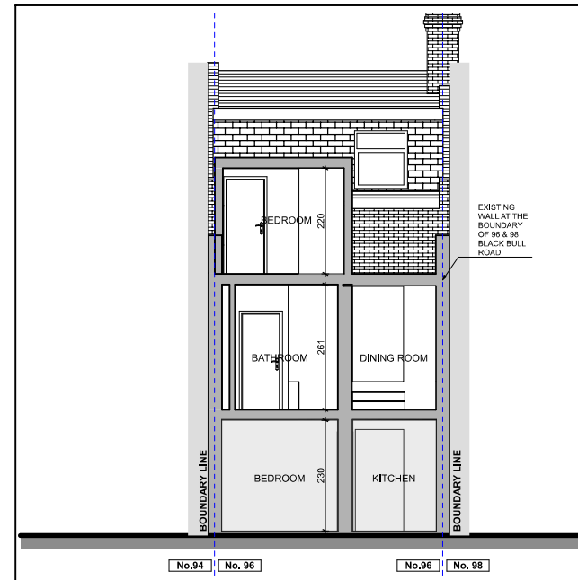
SECTION D-D
